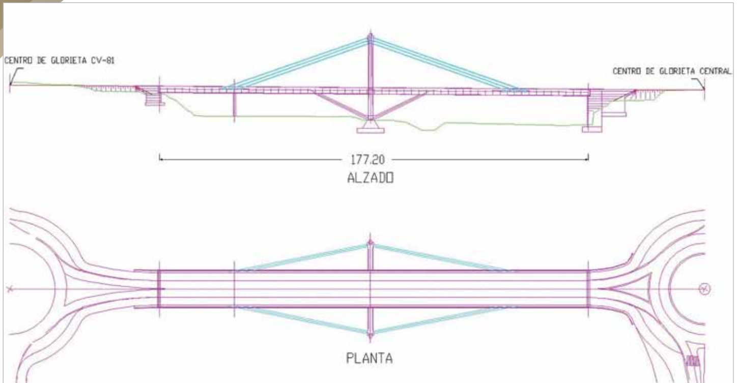
Planta i alçat del pont
